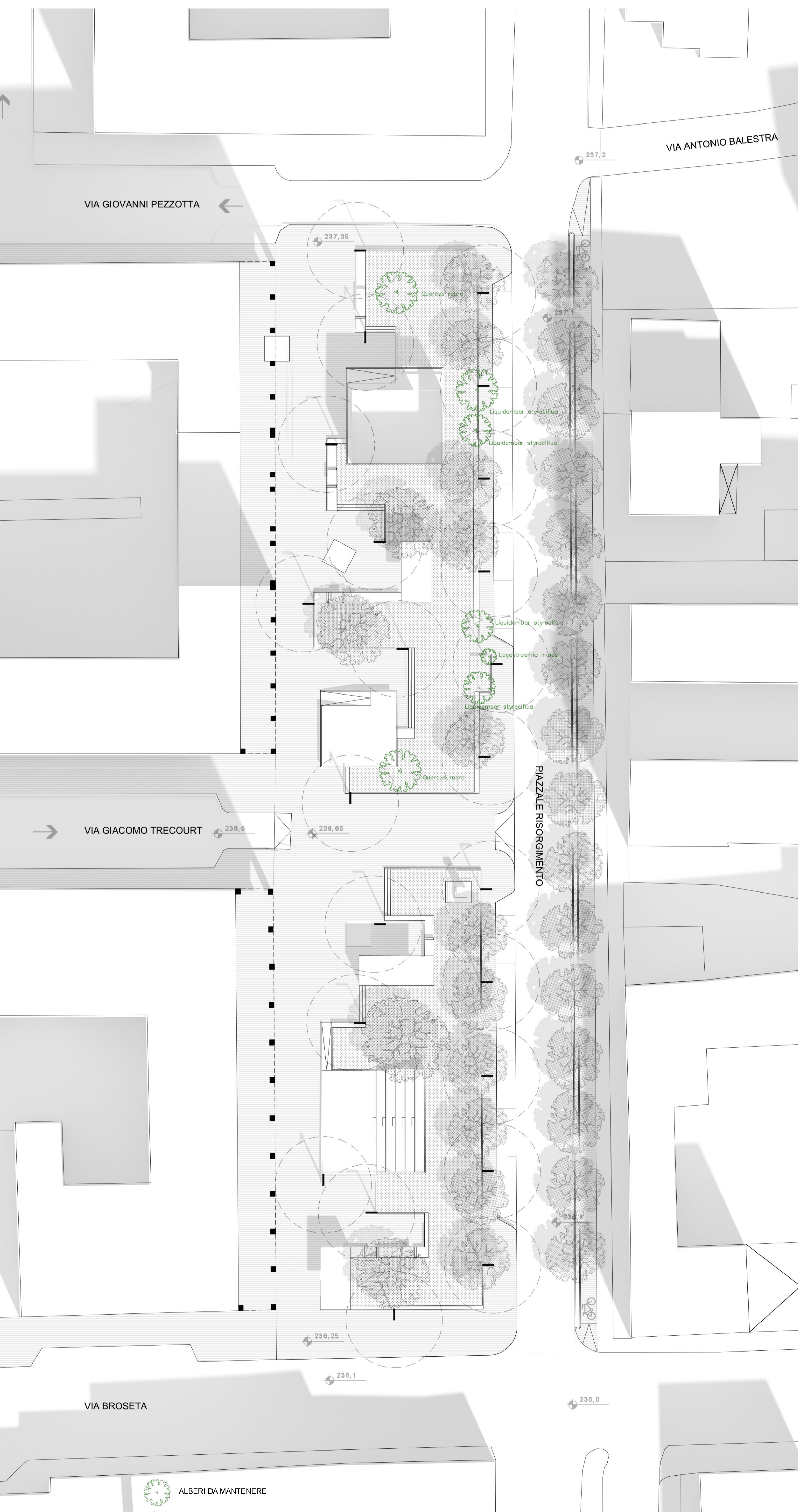
PLANIMETRIA GENERALE_SCALA 1:200
